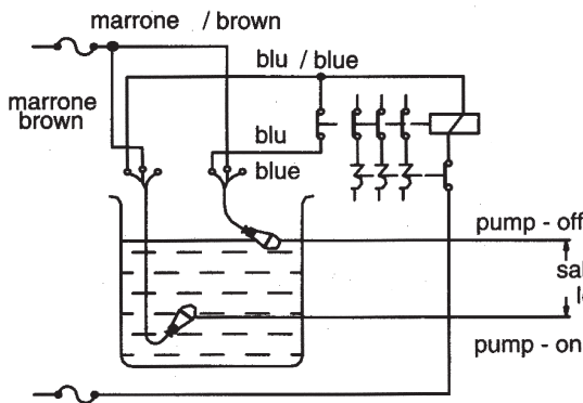
SCHEMA POMPA RIEMPIMENTO
